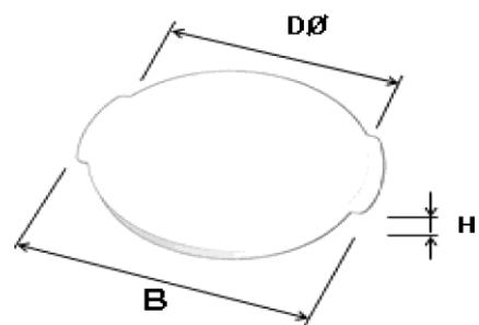
Schnappdeckel
